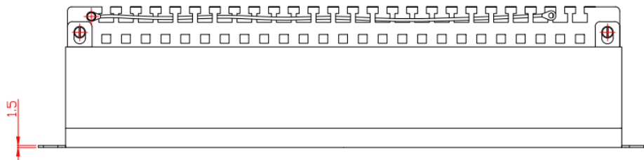
Вид сверху
