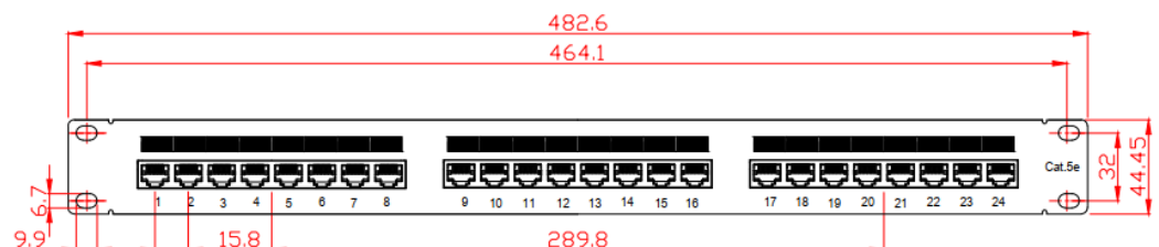
Вид спереди
