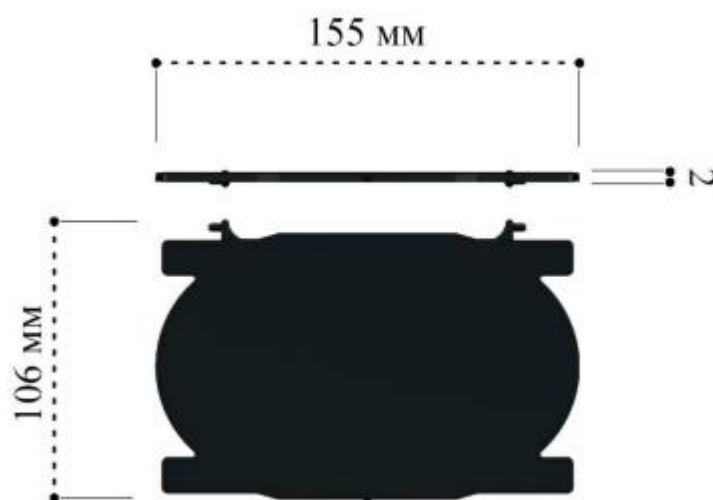
Крышка вид сверху
