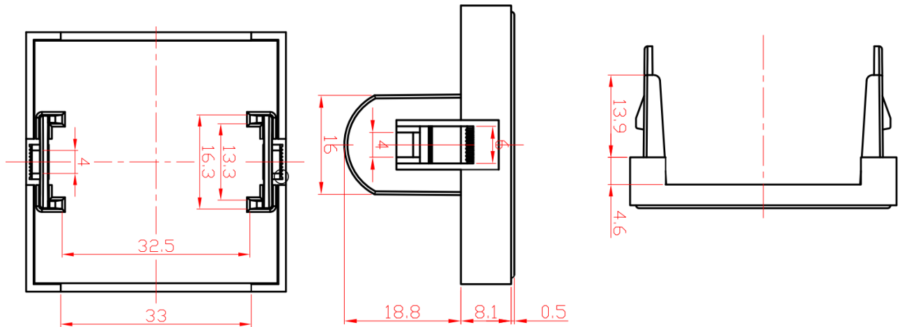
Вид сзади
