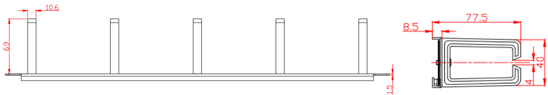
Вид спереди
