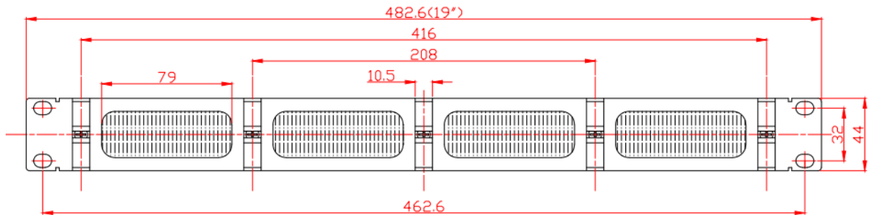
Вид спереди
