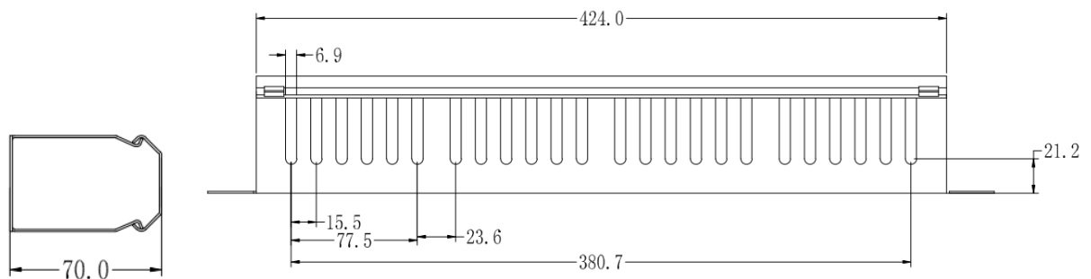
Вид сбоку
