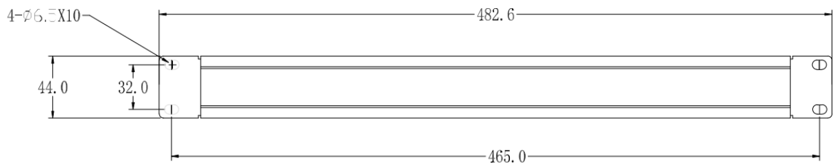
Вид спереди
