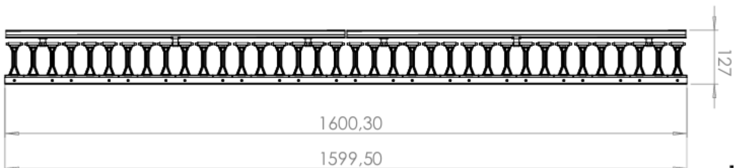
Вид сбоку
