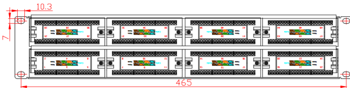
Вид сзади
