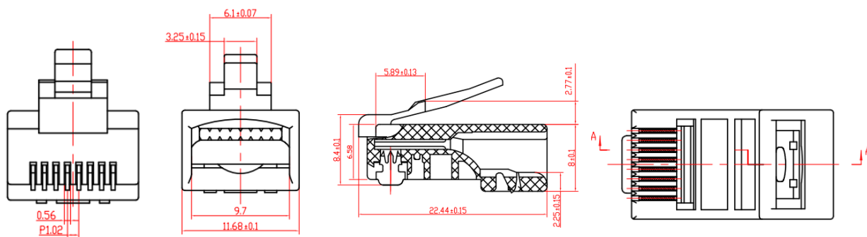
Вид спереди
