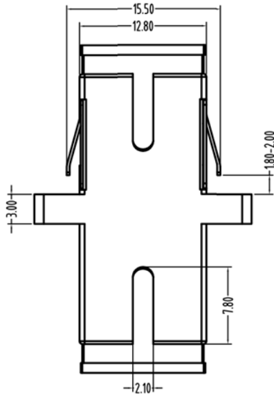
Вид сверху
