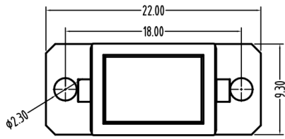
Вид спереди
